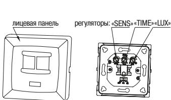
Рисунок 14 – Конструкция датчика движения ДД-031
