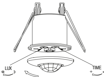
Рисунок 13 – Датчик движения ДД-301
